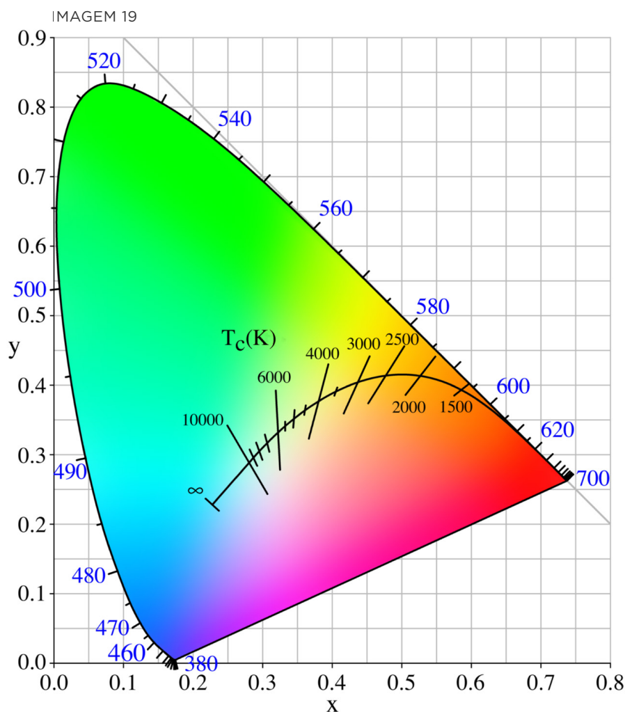
Curva de planck
